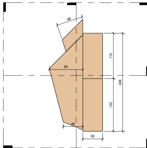
Elevation Top ⑦ 1 : 25
