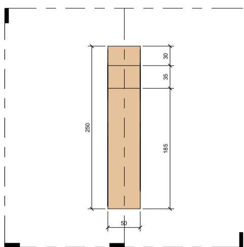
7 גב 1:25
