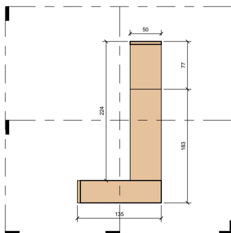
Elevation Right ⑥ 1 : 25
