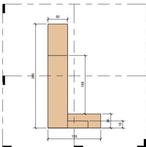
Elevation Back ④ 1 : 25
