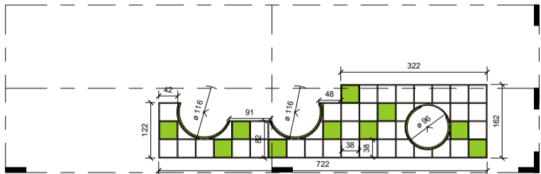
5 חזית 1 : 50
