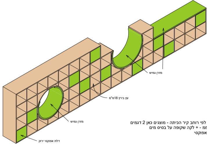
1 איזומטריה דגם 1
