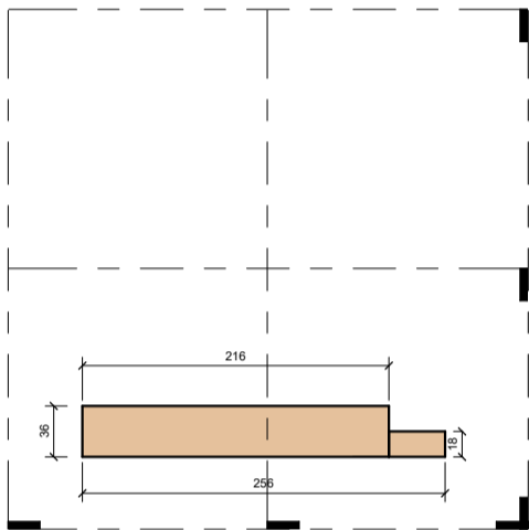
Detail Section B ③ 1 : 25
