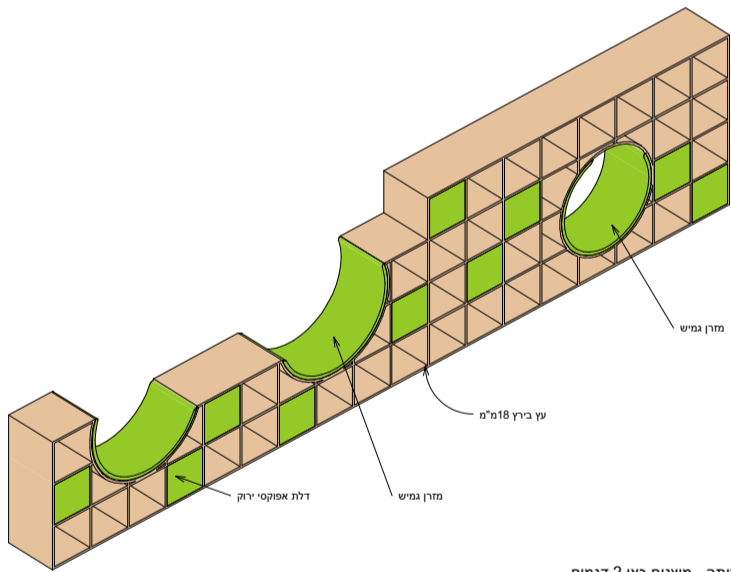
2 איזומטריה דגם 2
