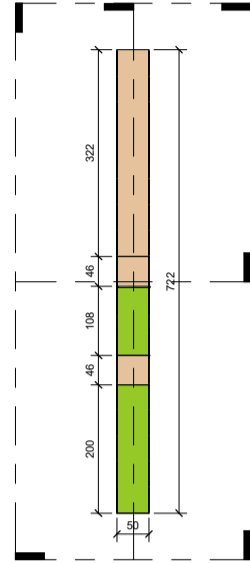
9 מבט עליון 1 : 50
