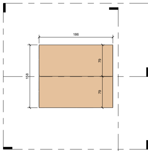
מבט עליון ③ 1 : 25
