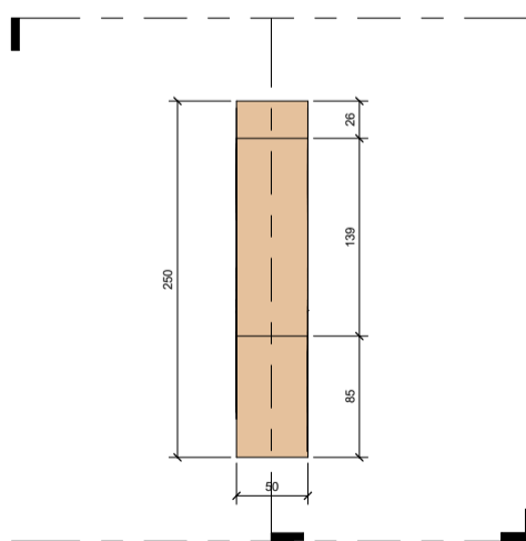
4 מבט על 1:25
